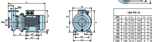
Fig.2 mit Drehstrommotor Baugröße 160-200
